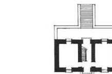
*H Plaisance. Πρόσοπος (1:200), Κάτοπος (1:400).
