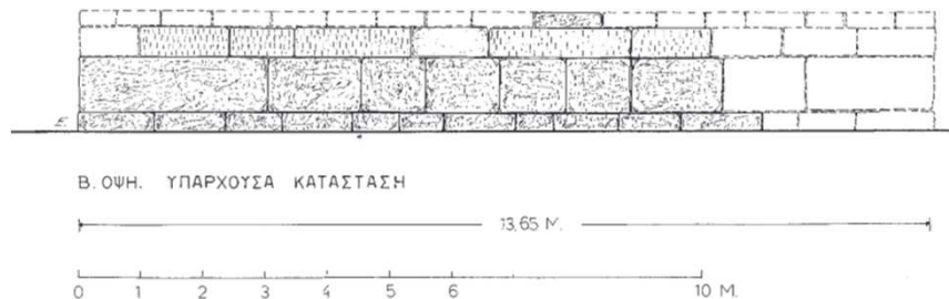
Εικ. 7. Σχέδιο της υπάρχουσας κατάστασης της πρόσοψης του ταφικού περιβόλου (σχέδ. Κ. Καζαμιάκη).
