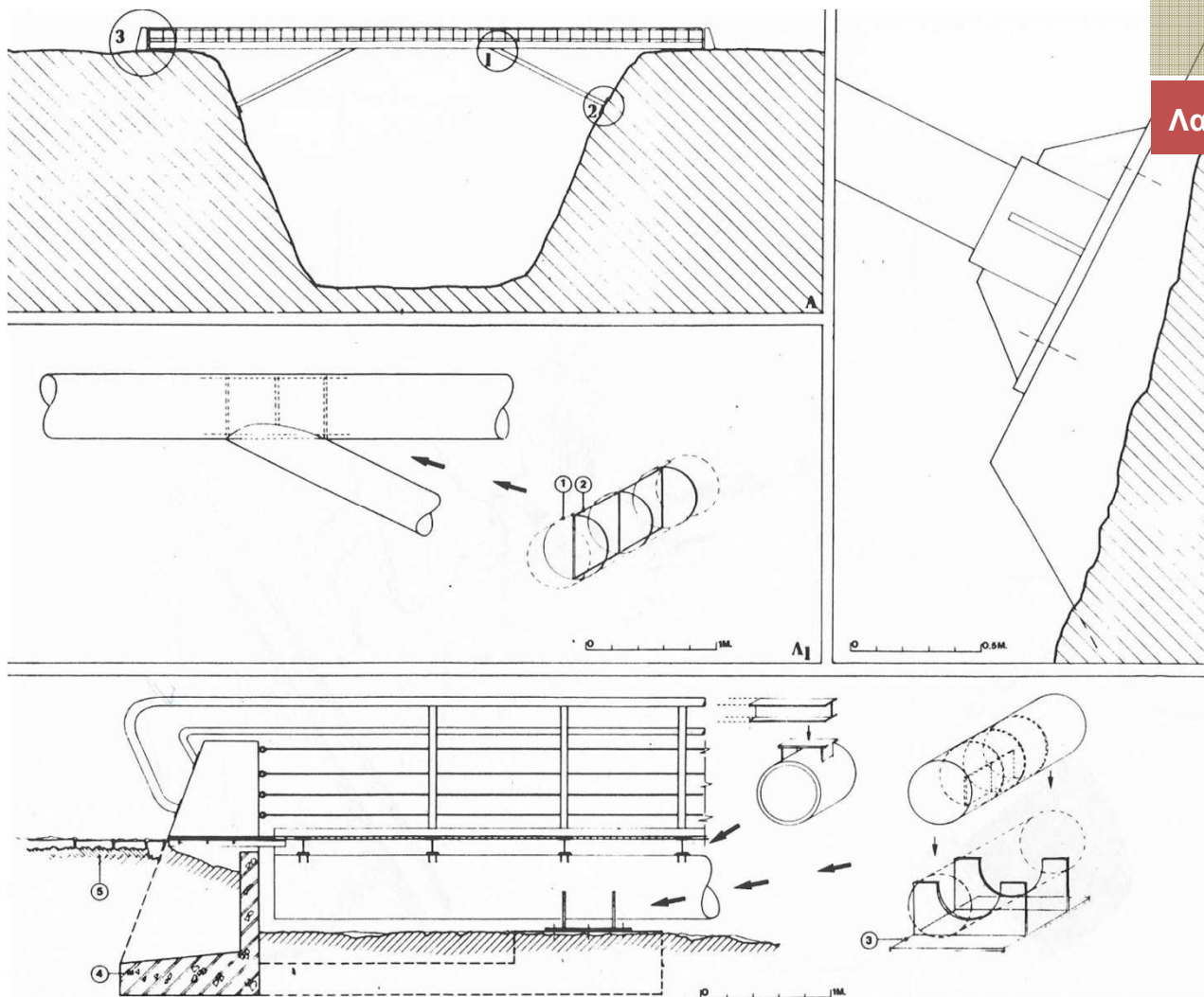
1. ΚΑΤΑΣΚΕΥΗ ΠΕΖΟΓΕΦΥΡΑΣ
